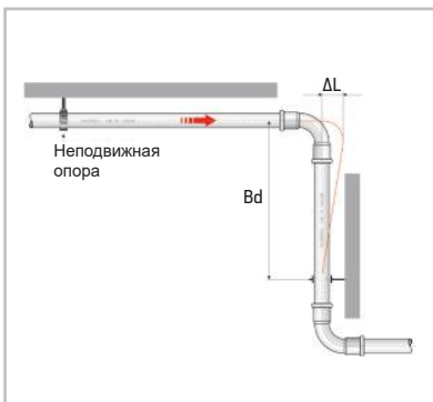
Рис. 46. Z-образный компенсатор.
