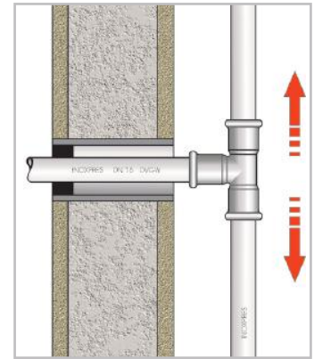
Рис. 45с. Создание компенсационных зазоров.
