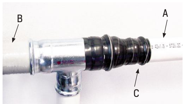
Рис. 39. Материалы для защиты от внешней коррозии: А. Труба с защитой из полипропилена; В. Покраска праймером; С. Защита бутаноловой клейкой лентой.
