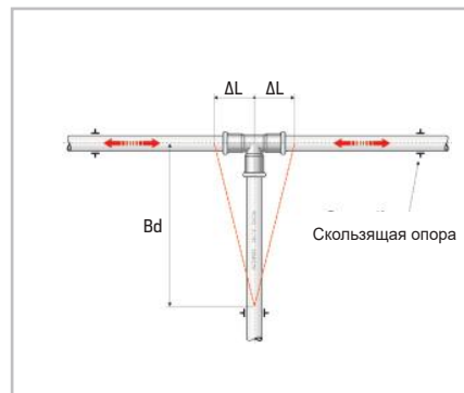
Рис. 47. Т-образный компенсатор.
