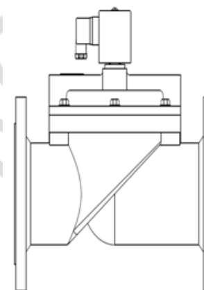
Рисунок 1. Устройство
